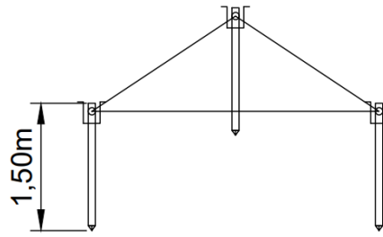
Εικόνα 50: Τρίγωνο γείωσης
