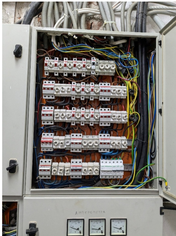
Ηλεκτρολογικός πίνακας 25
