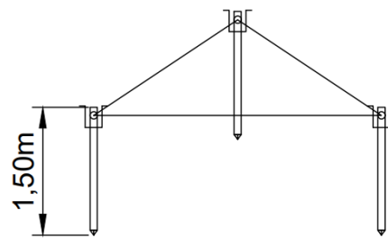
Εικόνα 50: Τρίγωνο γείωσης
