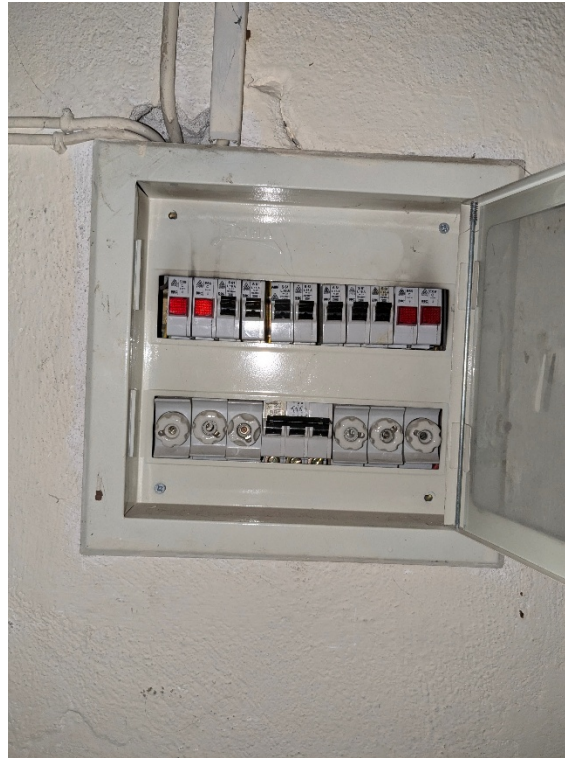
Ηλεκτρολογικός πίνακας 17
