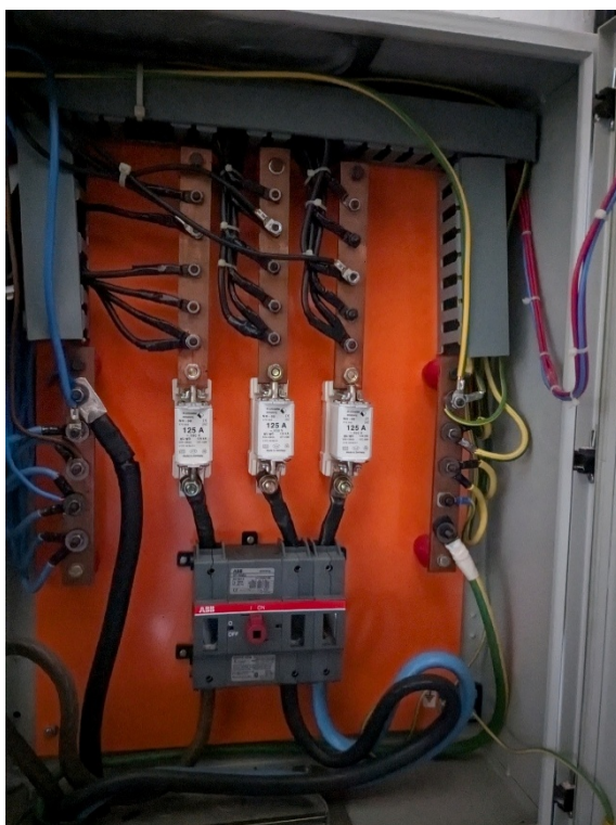
Ηλεκτρολογικός πίνακας 24
