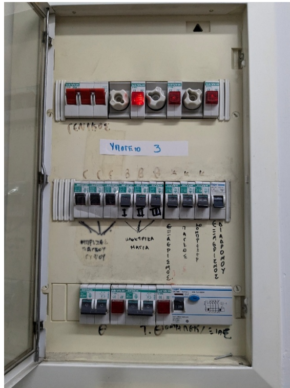
Ηλεκτρολογικός πίνακας 19
