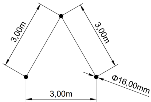
Εικόνα 49: Τρίγωνο γείωσης
