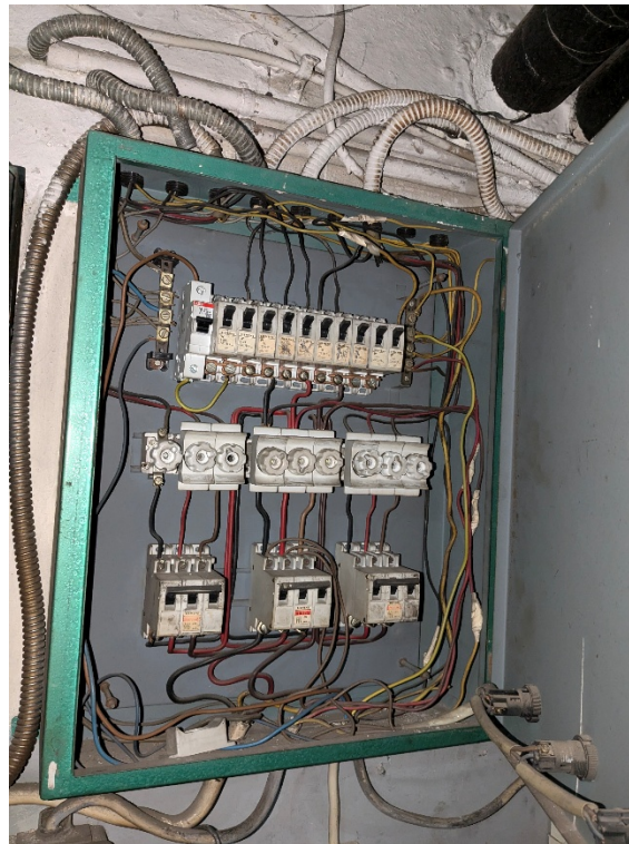
Ηλεκτρολογικός πίνακας 19
