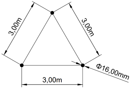
Εικόνα 49: Τρίγωνο γείωσης
