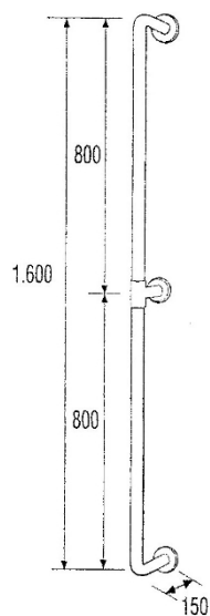
Κάθετος χειρολισθήρας με 3 σημεία στήριξης στον τοίχο.
