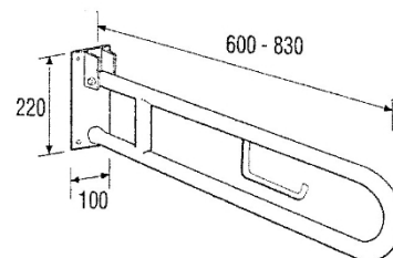
Μπάρα στήριξης με χαρτοθήκη
