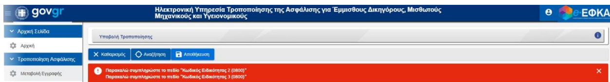
Εικόνα 2 Μήνυμα Σφάλματος 2
