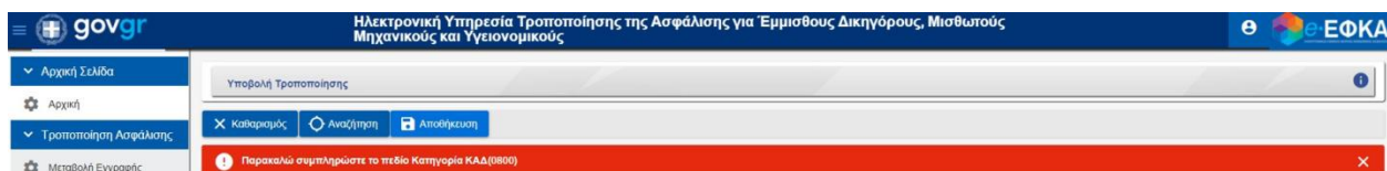
Εικόνα 1 Μήνυμα Σφάλματος 1
